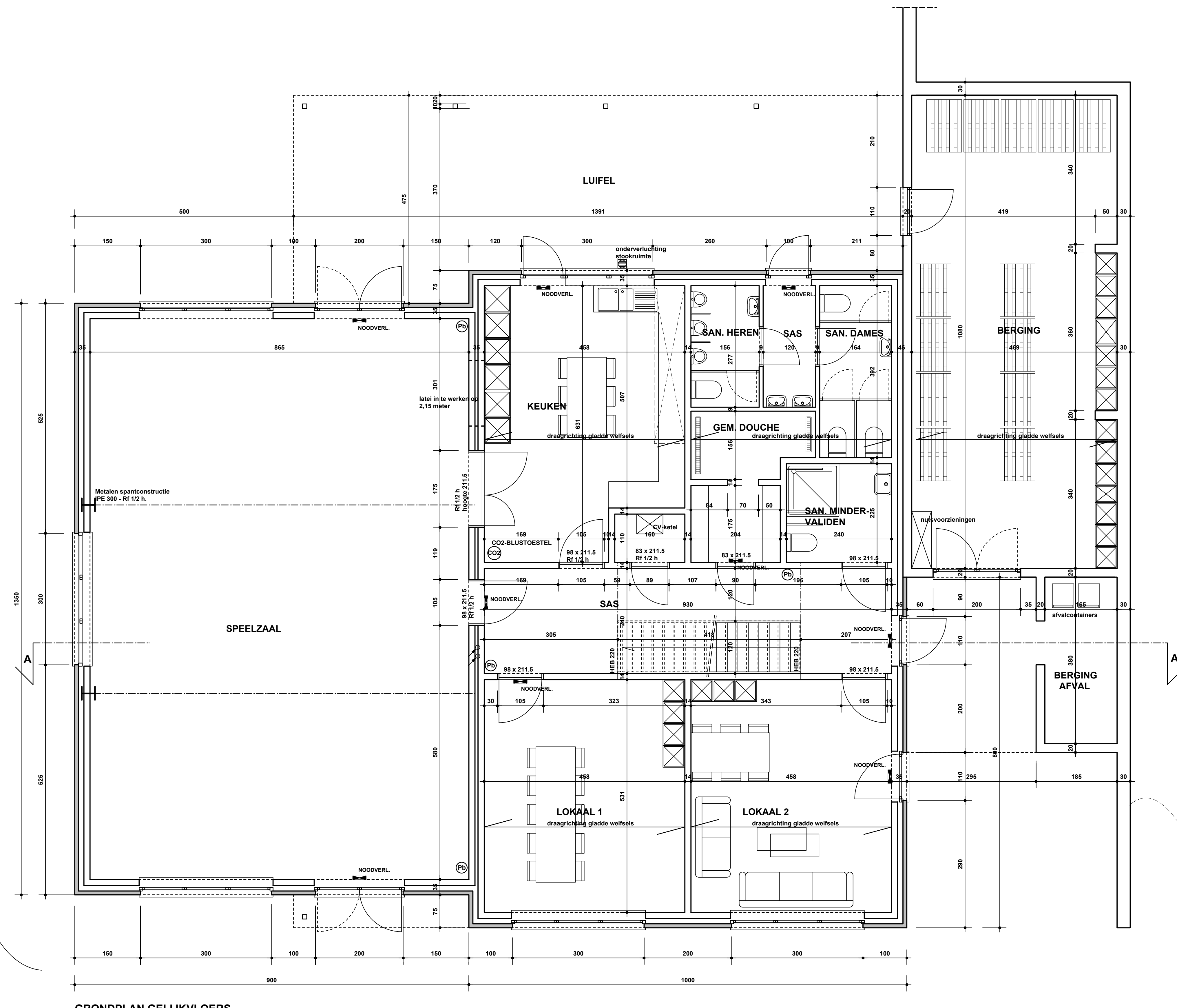
GRONDPLAN GELIJKVLOERS
