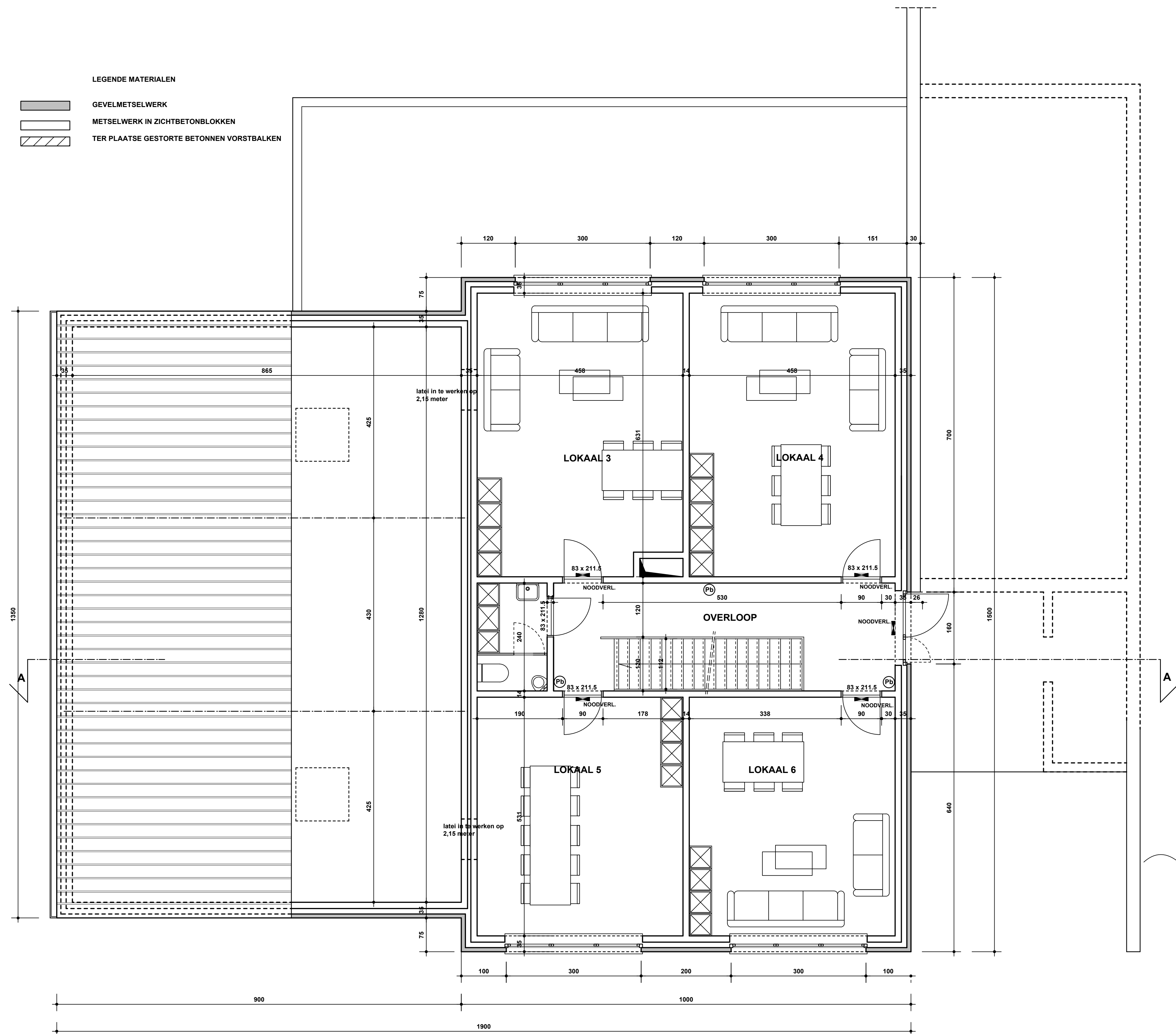
GRONDPLAN VERDIEPING
