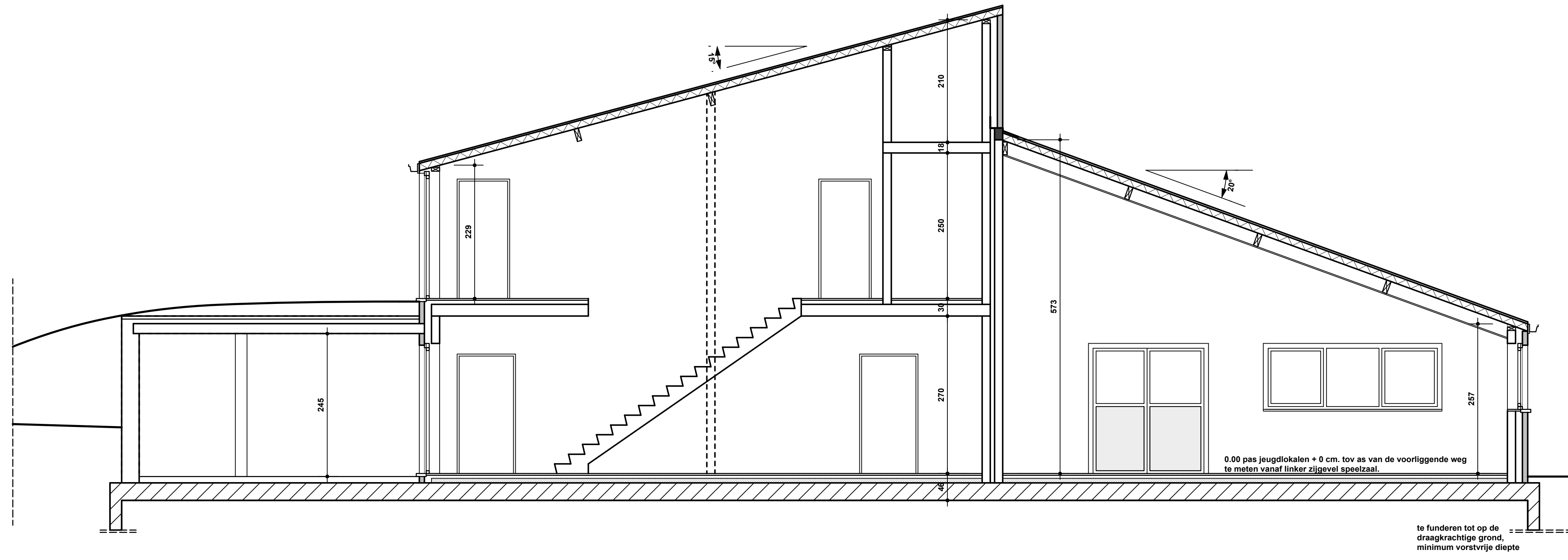
SNEDE AA
