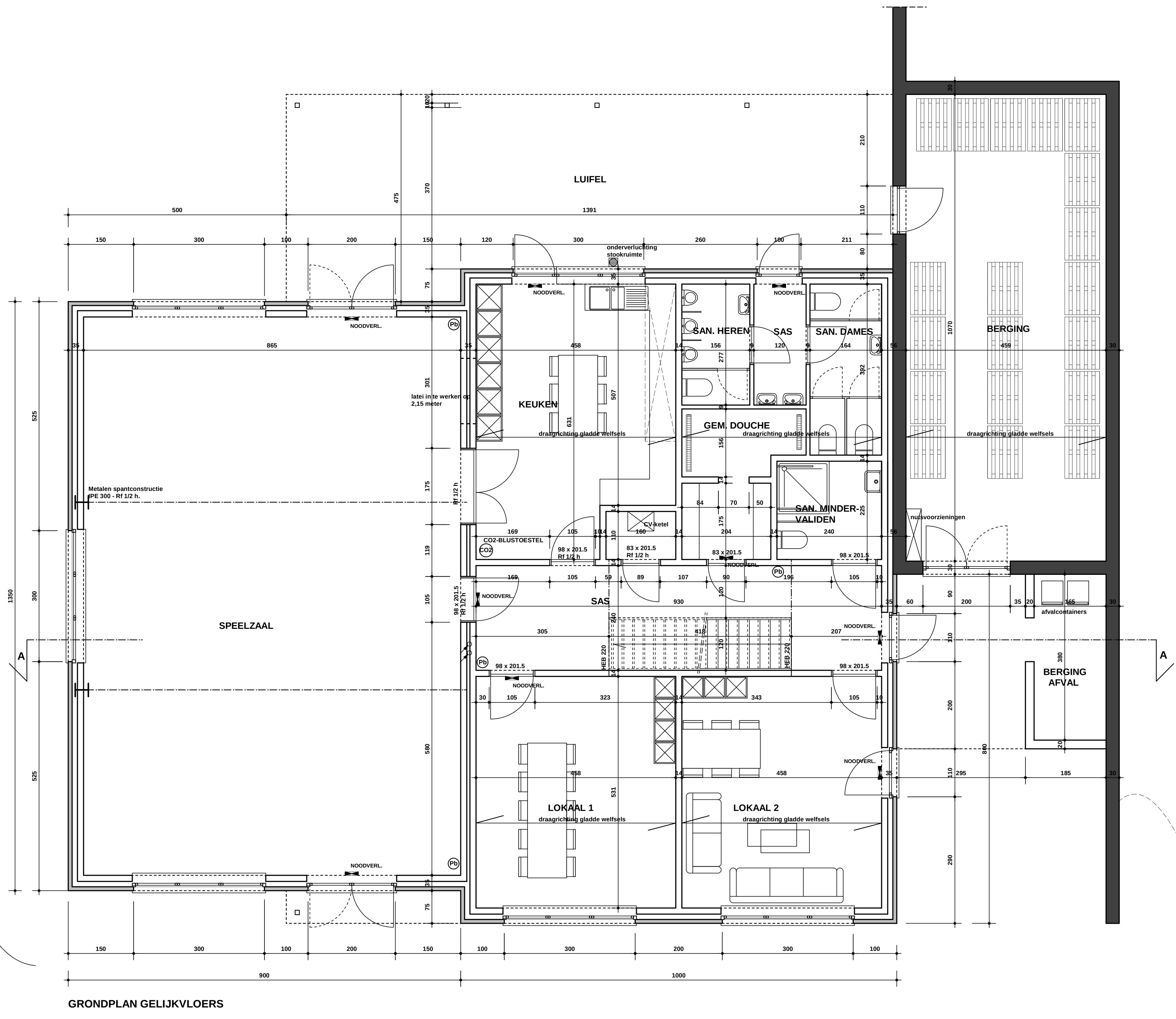
GRONDPLAN GELIJKVLOERS
