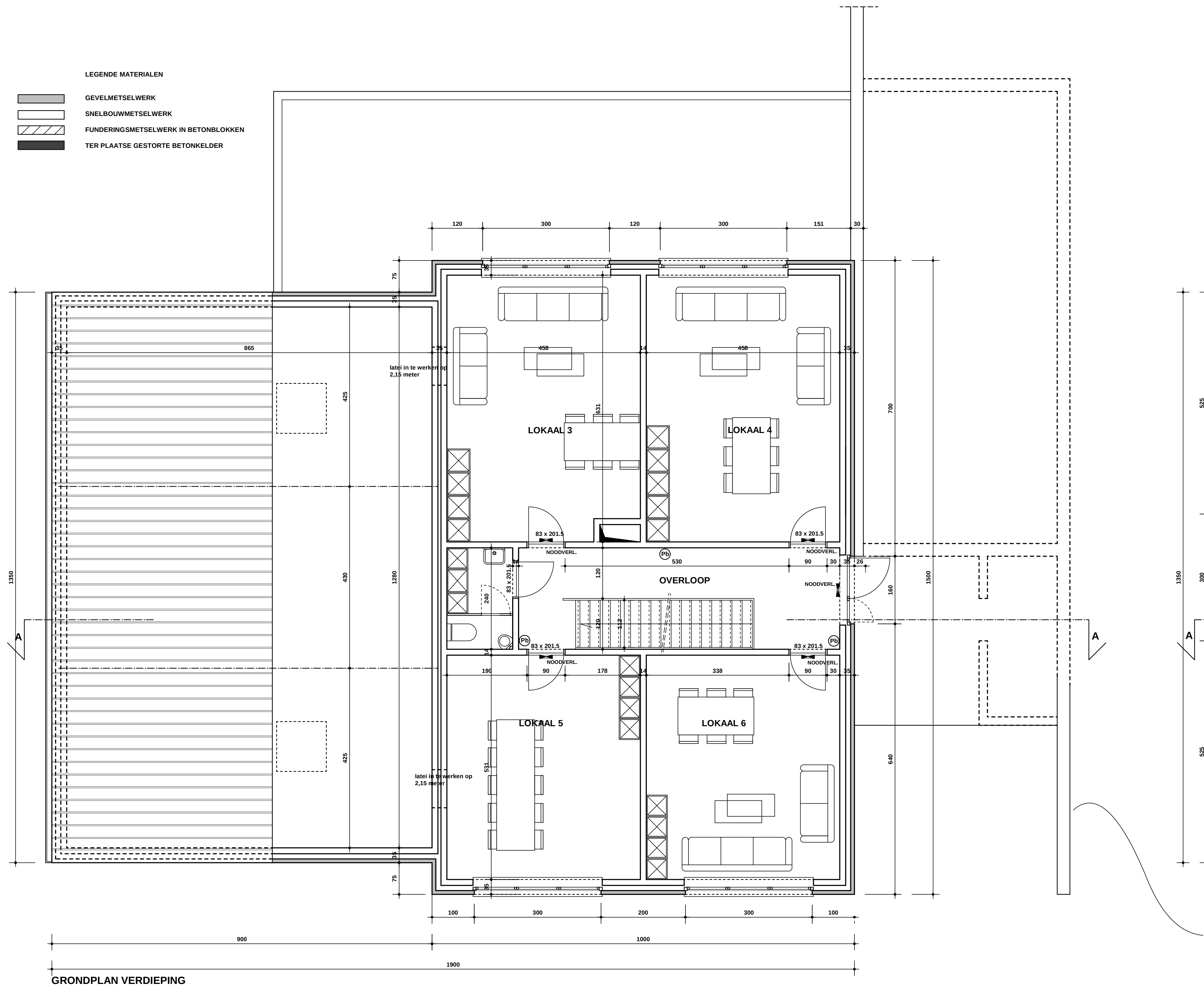
GRONDPLAN VERDIEPING
