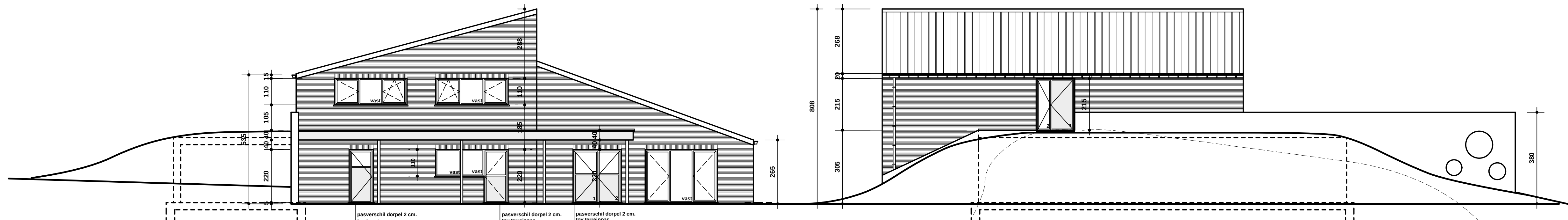
ACHTERGEVEL schaal 1 / 100
