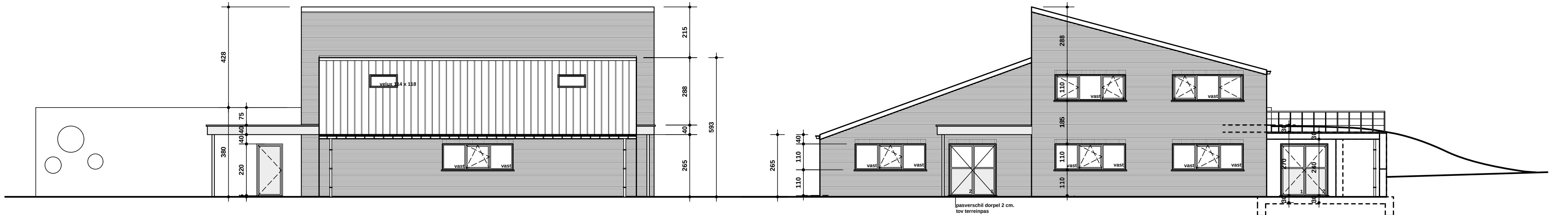
ZIJGEVEL LINKS schaal 1 / 100
